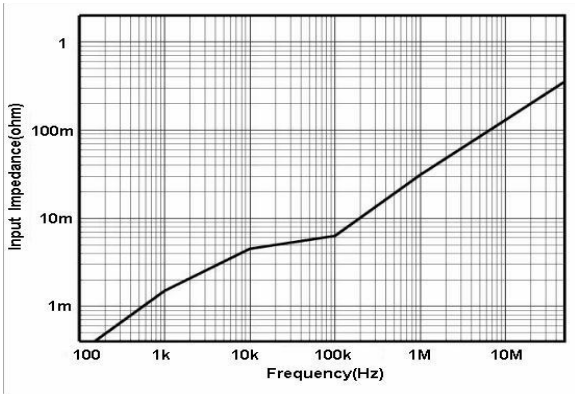
图 3.a HCP8030 输入阻抗 VS 频率曲线
