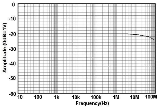
图 4 HCP8050 幅频曲线
