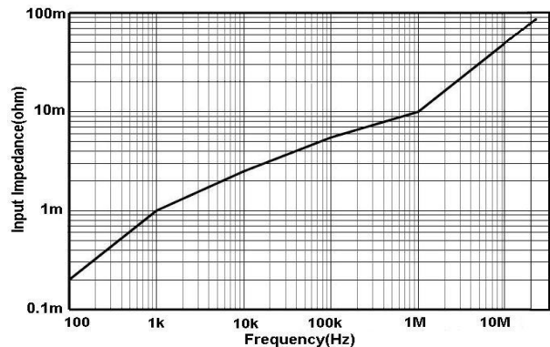
图 12.b HCP8150A 输入阻抗 VS 频率曲线
