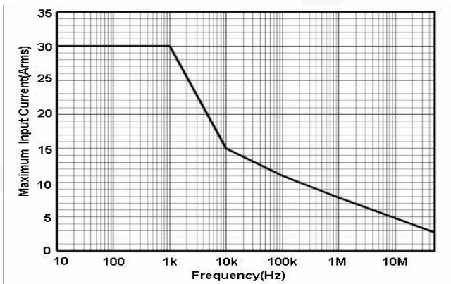
图 2.a HCP8030 最大测量电流 VS 频率曲线
