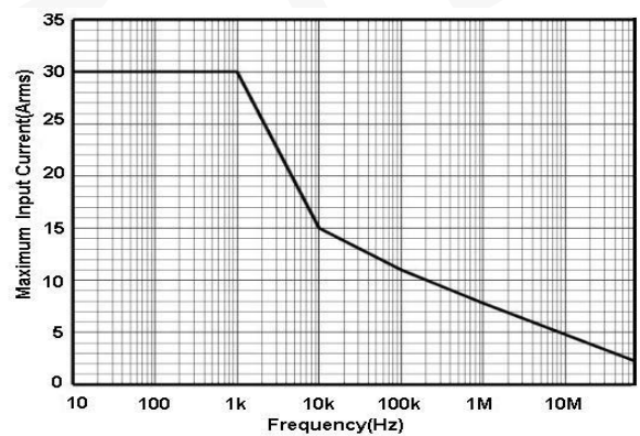
图 2.b HCP8030C 最大测量电流 VS 频率曲线
