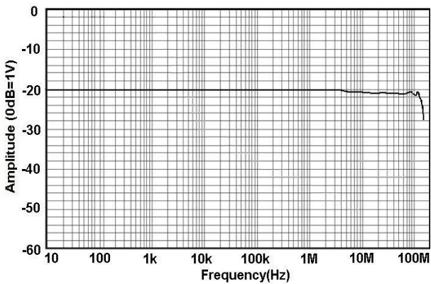
图 1.c HCP8030D 幅频曲线
