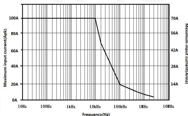
图 3 最大电流 VS 频率特性曲线
