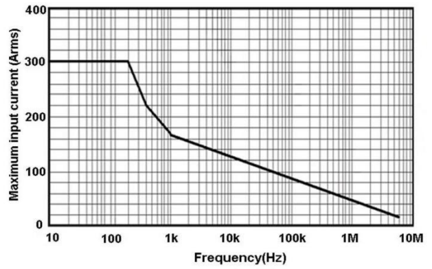
图 11.a HCP8300 最大测量电流 VS 频率曲线 (超过该曲线所示最大电流连续使用会导致探头烧毁)
