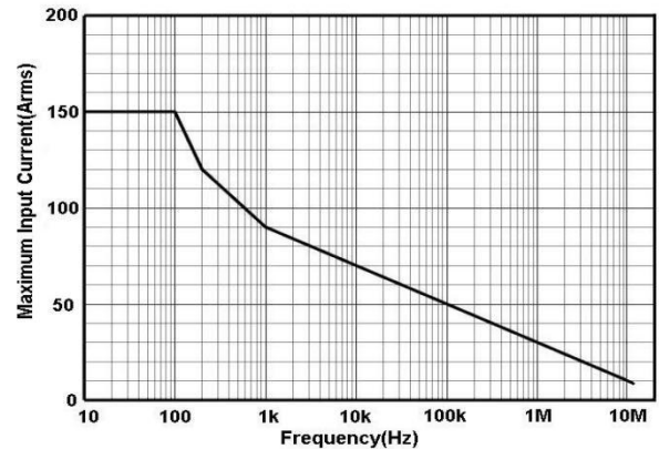
图 8.a HCP8150 最大测量电流 VS 频率曲线 (超过该曲线所示最大电流连续使用会导致探头烧毁)
