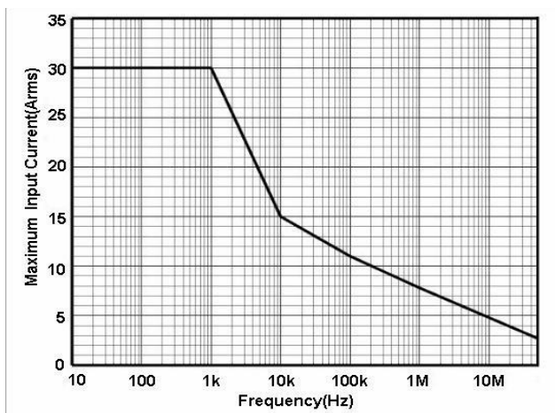
图 2.a HCP8030 最大测量电流 VS 频率曲线
