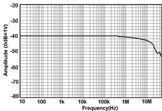
图 10.a HCP8300 幅频曲线
