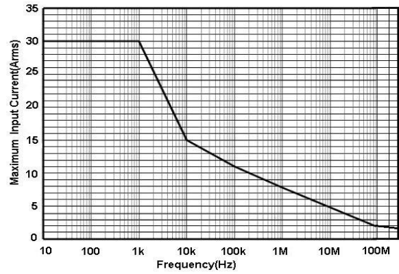
图 2.d HCP8030H 最大测量电流 VS 频率曲线 (超过该曲线所示最大电流连续使用会导致探头烧毁)
