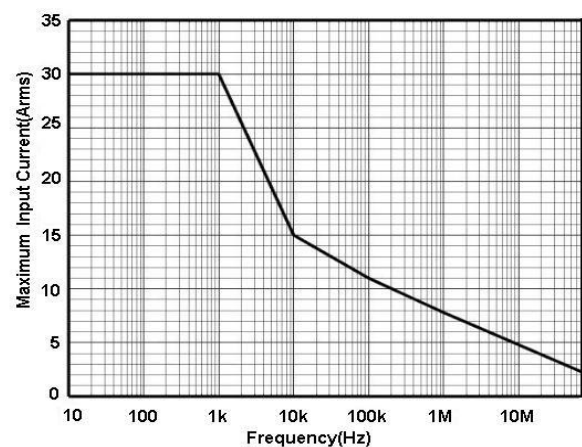
图 2.b HCP8030C 最大测量电流 VS 频率曲线
