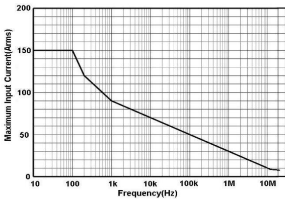
图 8.b HCP8150A 最大测量电流 VS 频率曲线 (超过该曲线所示最大电流连续使用会导致探头烧毁)
