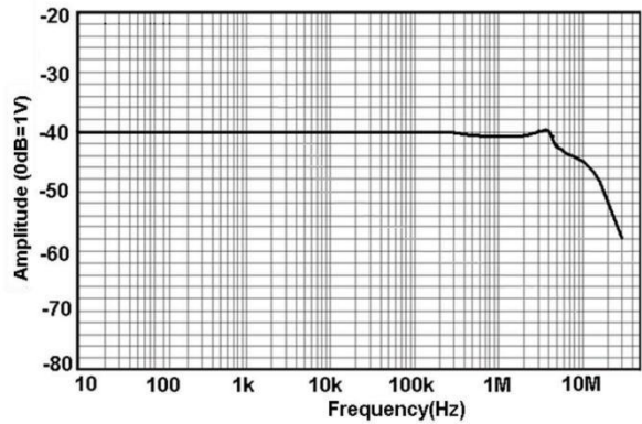
图 13 HCP8500 幅频曲线
