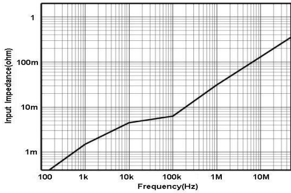
图 6 HCP8050 输入阻抗 VS 频率曲线
