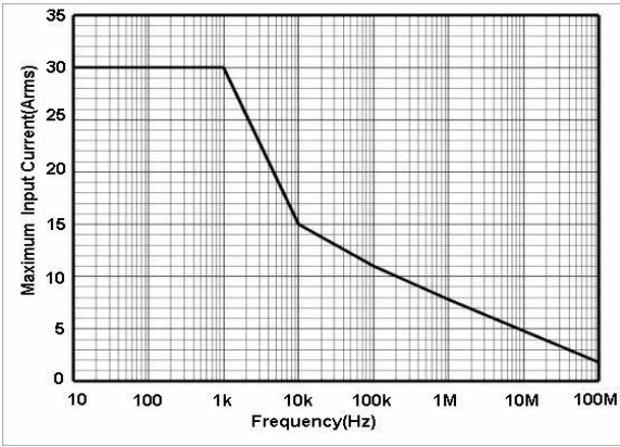
图 2.c HCP8030D 最大测量电流 VS 频率曲线 (超过该曲线所示最大电流连续使用会导致探头烧毁)
