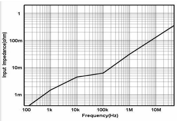
图 3.a HCP8030 输入阻抗 VS 频率曲线
